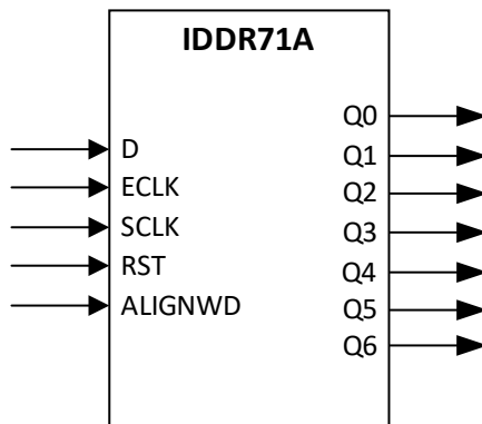
Figure 5.12. IDDR71A Ports
