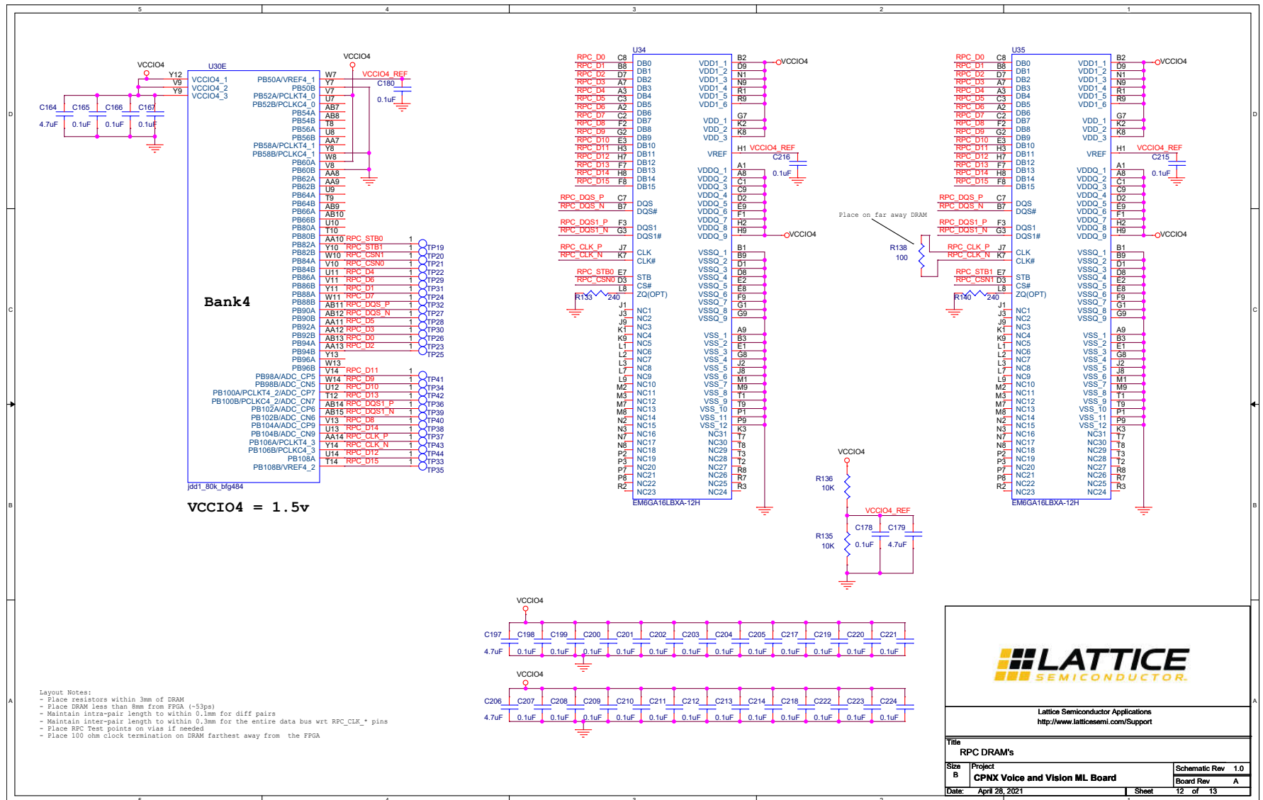
Figure A.12. RPC DRAMs
