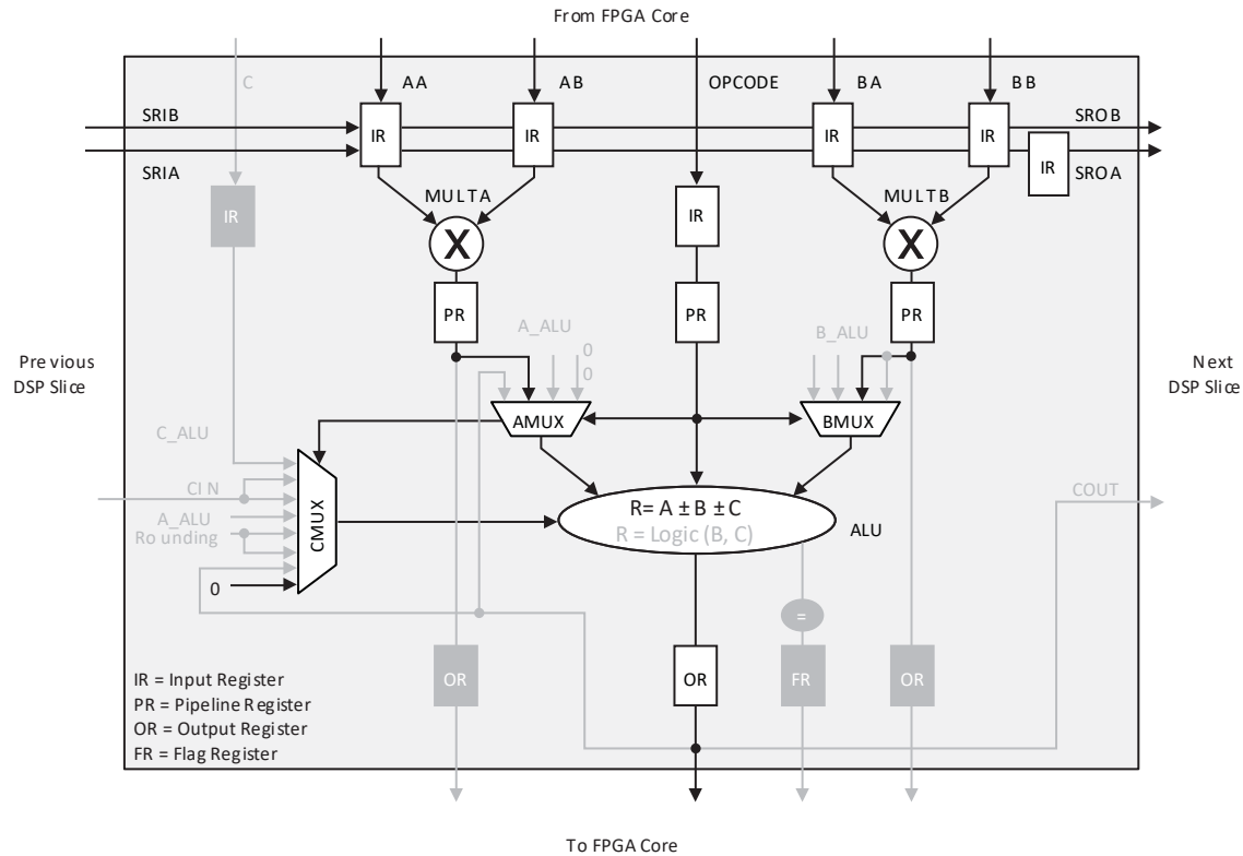
Figure 3.28. MULTADDSUB
