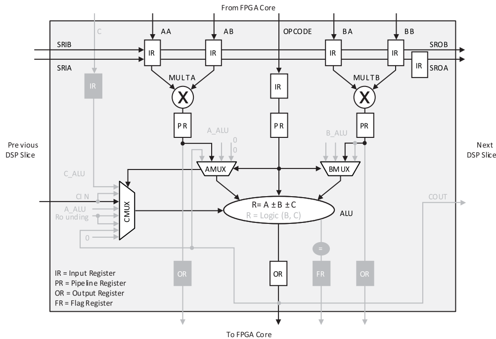
Figure 3.30. MULTADDSUBSUM Slice 1
