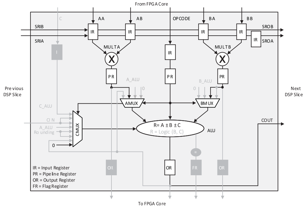
Figure 3.29. MULTADDSUBSUM Slice 0
