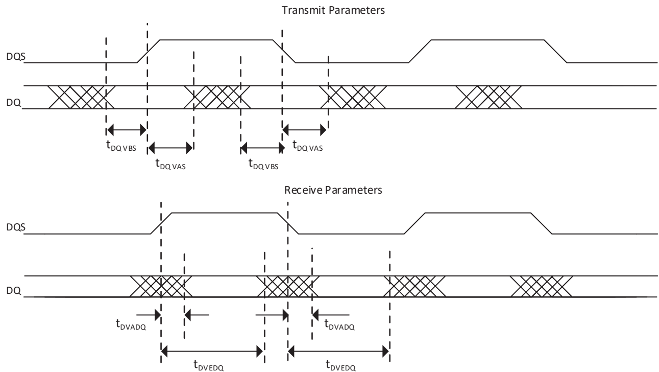
Figure 4.7. DDR/DDR2/DDR3 Parameters
