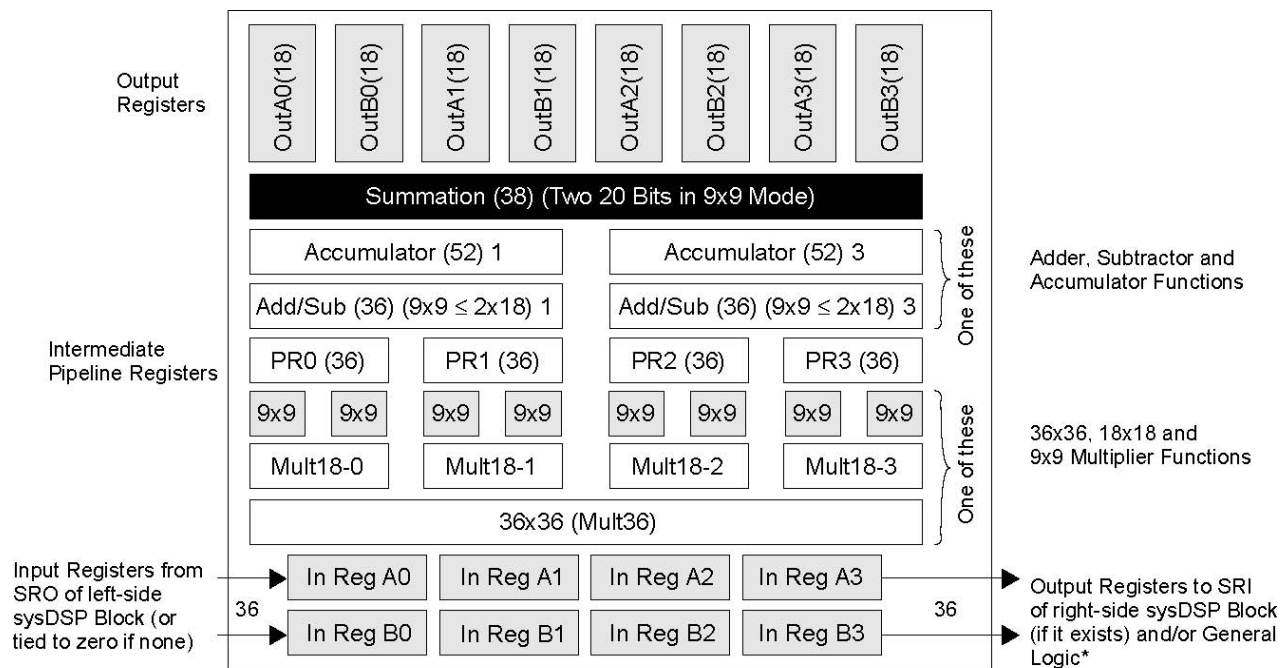
図12-1 LatticeECP2/M sysDSPブロック図
