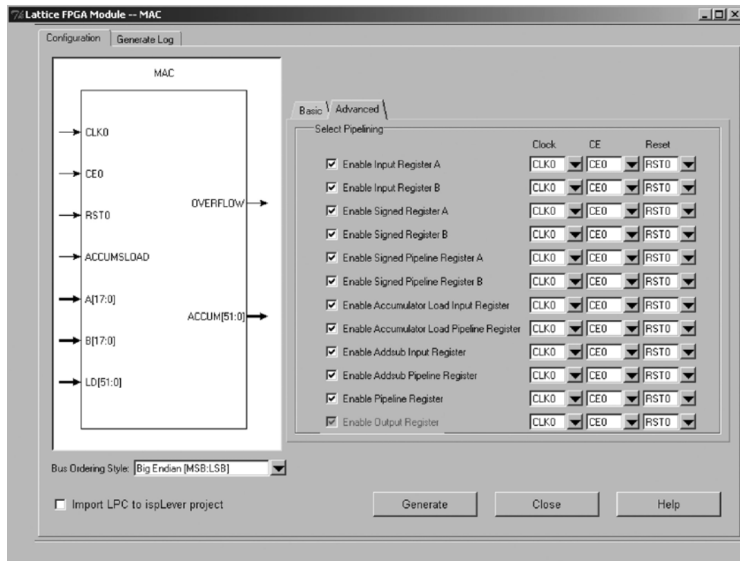
図12-5 MACモードのアドバンスド・セットアップ
